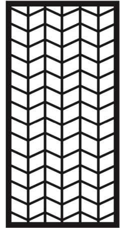
Quiver ≈ 62% Vis
