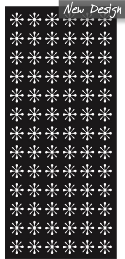
Daisy ≈ 14% Vis
